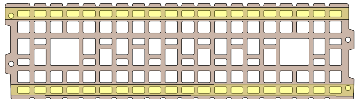
4. Breng de lijmrillen aan op schone en stofvrije blokken (2 horizontale rillen per steen op de wandrijen grenzend aan de buitenzijde)
